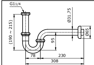
Bộ thoát thải chữ P (L=308mm) TVLF403
