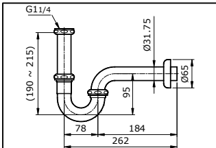
Bộ thoát thải chữ P (L=262mm) TVLF402
