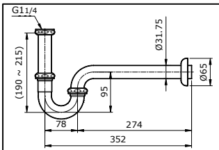
Bộ thoát thải chữ P (L=352mm) TVLF404
