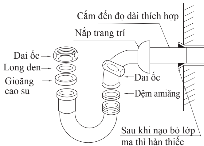
Sơ đồ lắp đặt phụ kiện thoát nước
