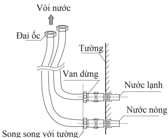
Sơ đồ lắp đặt phụ kiện cấp nước
